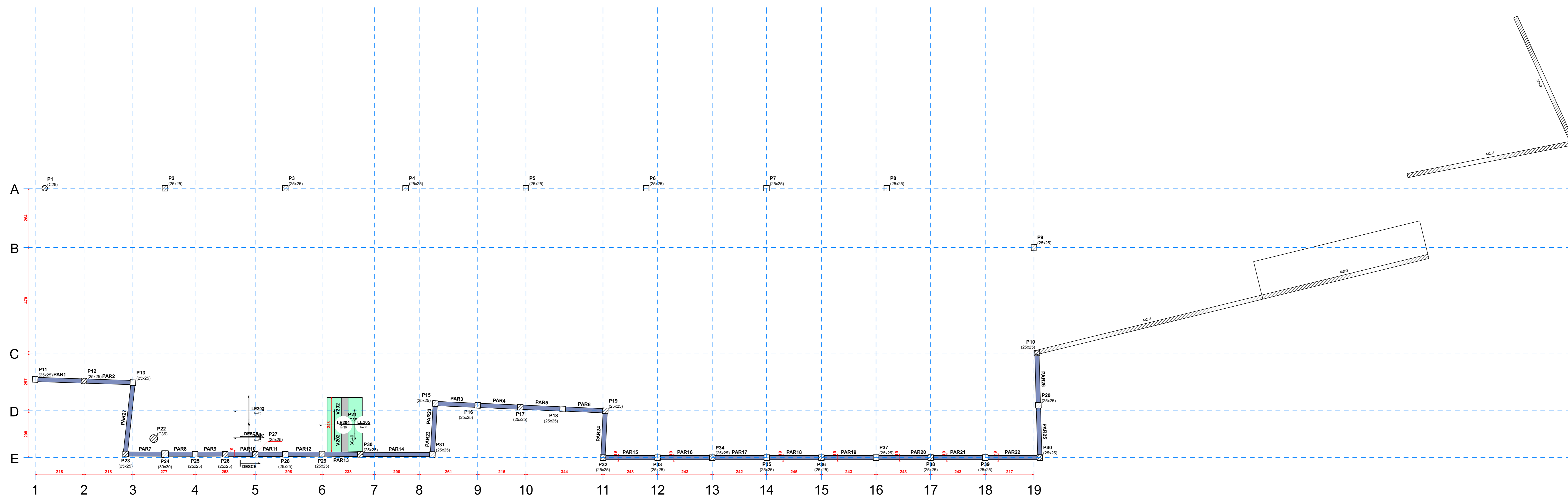
FORMA INTERMEDIÁRIA DO PAVIMENTO TOPO RAMPA (NÍVEL 53354)
