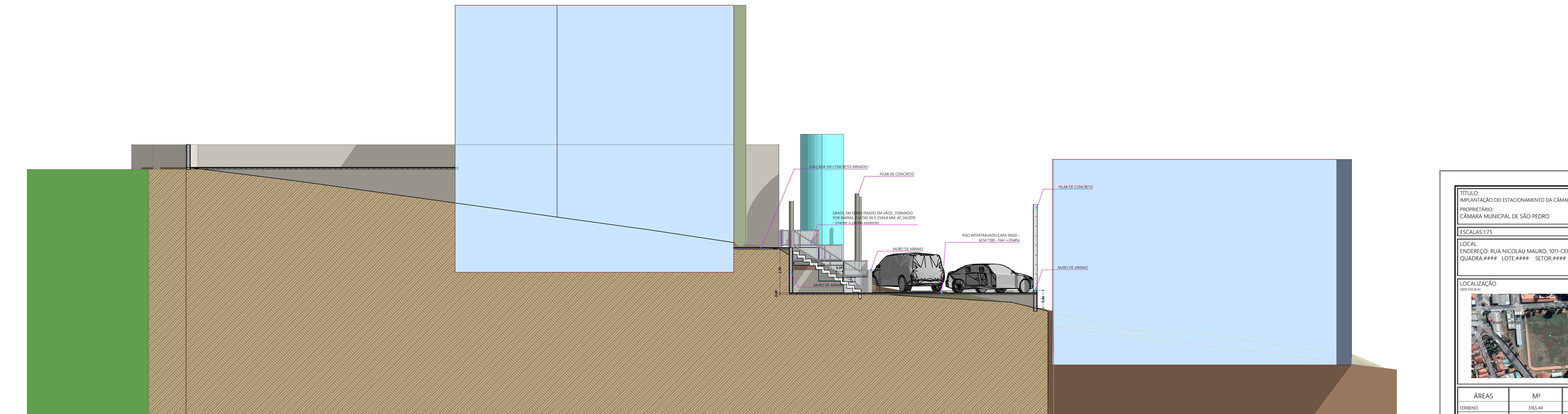
C-02 CORTE 1:75
